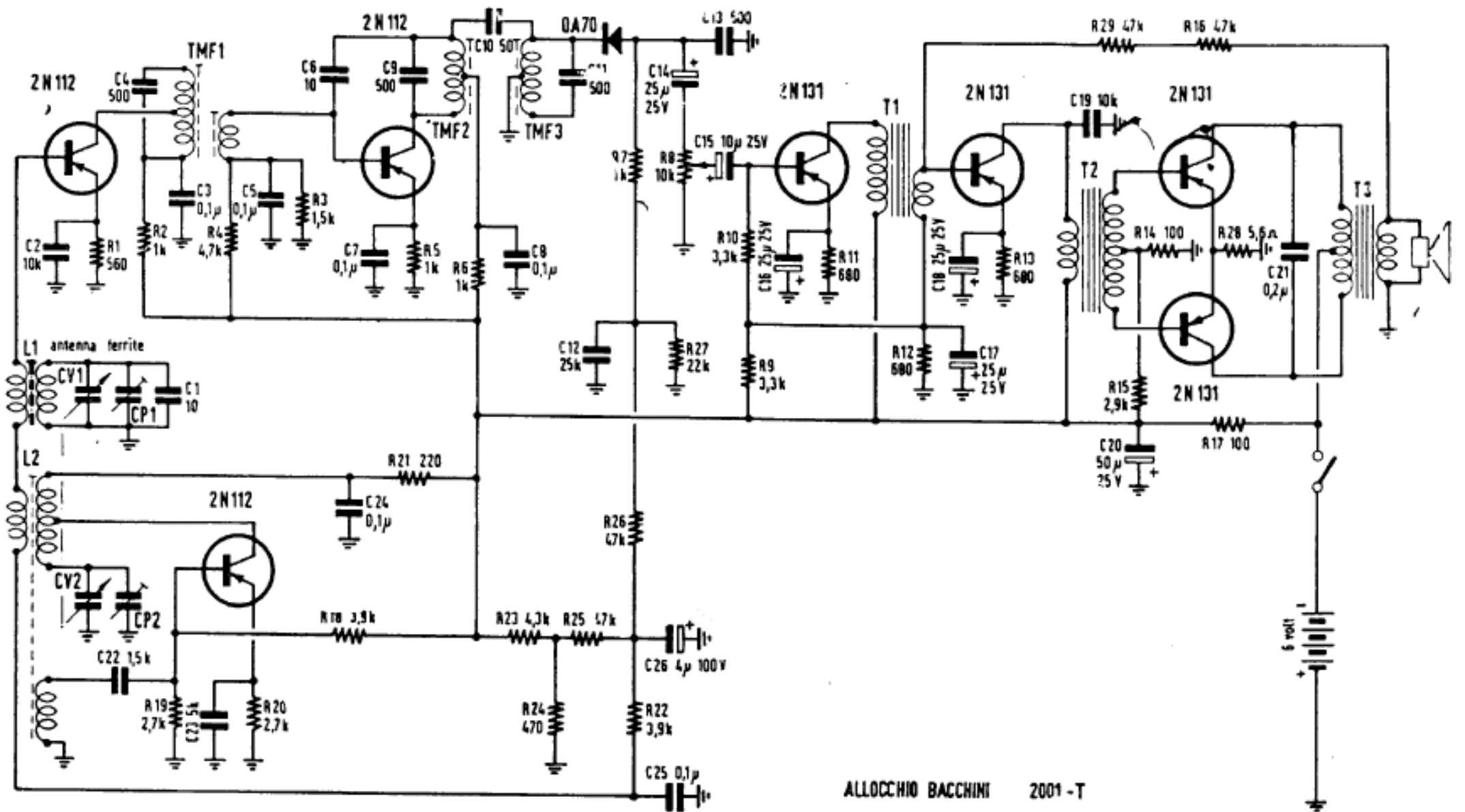
SCHEMA ELETTRICO DEL RADIORICEVITORE A TRANSISTORI ALLOCCIO BACCHINI MOD. 2001-T
